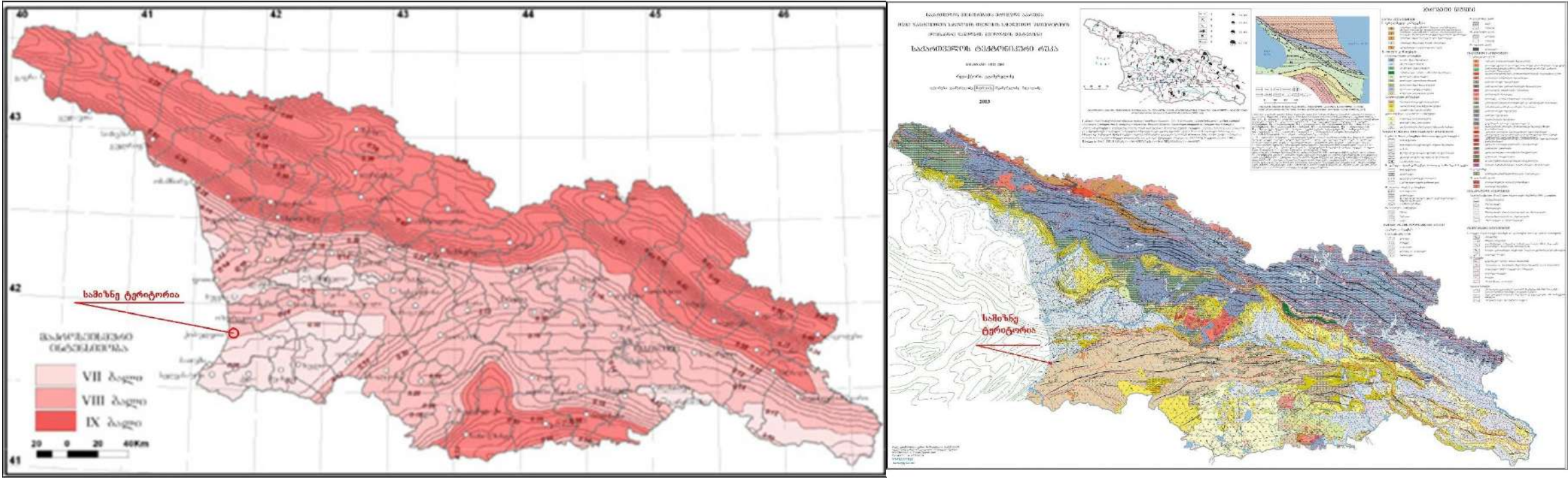
სეისმიური საშიშროების რუკა - მაქსიმალურ ჰორიზონტალურ აჩქარებასა და ბალებში
