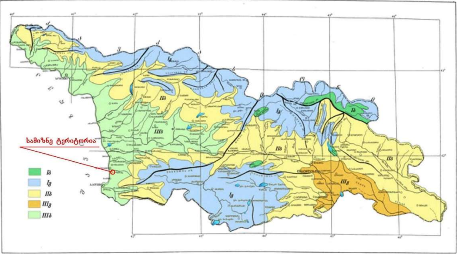
საქართველოს ტერიტორიის სამშენებლო კლიმატური დარაიონება
