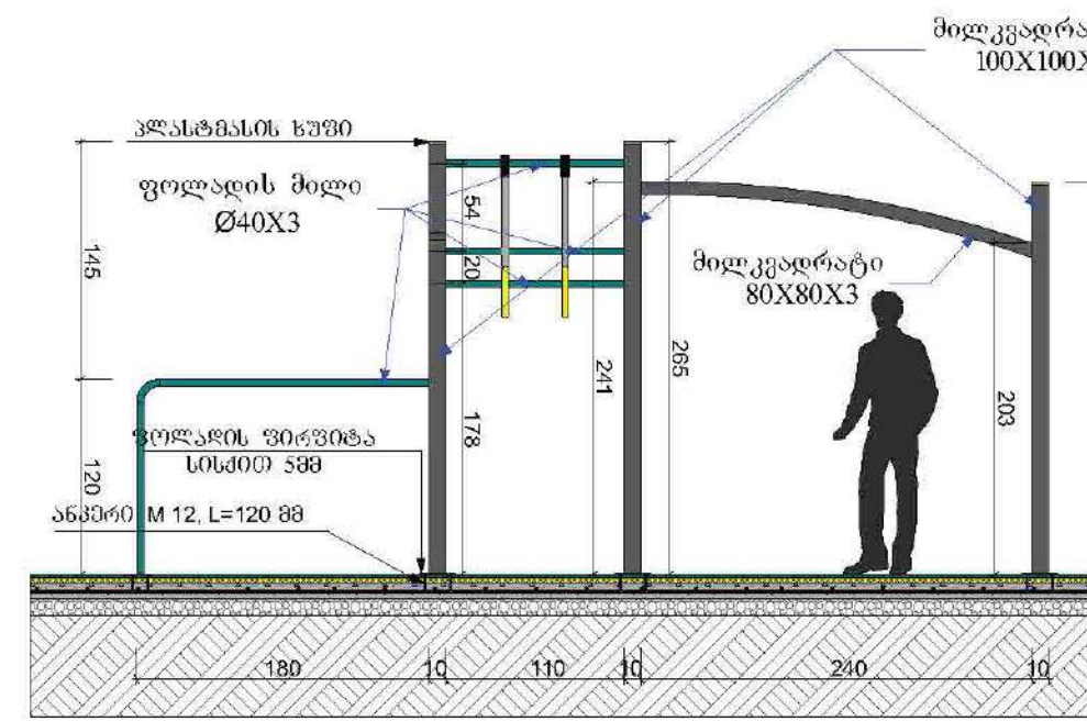
ხელი 2 მ 1:50
