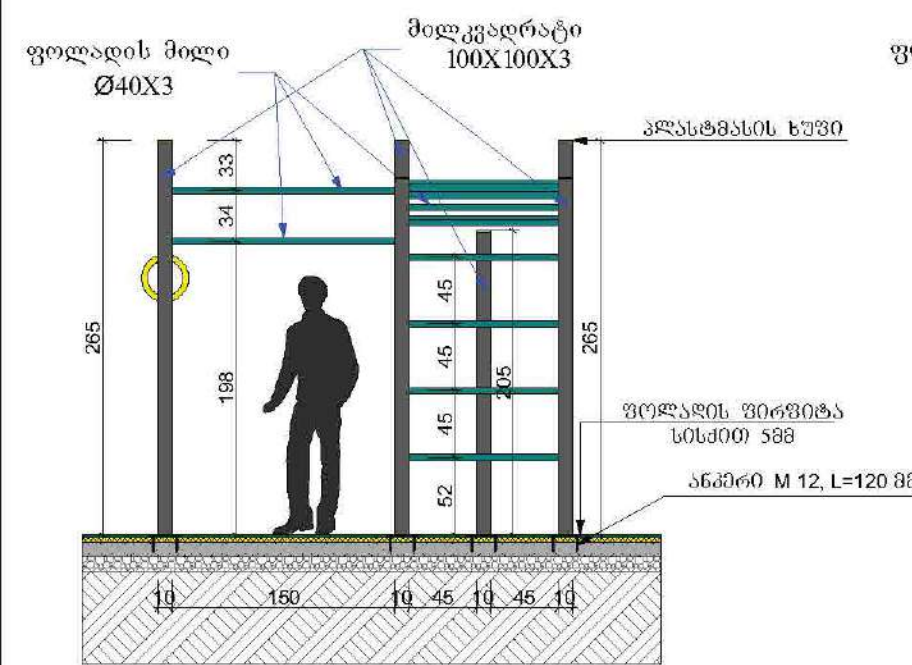
ხელი 3 მ 1:50
